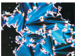
偏光顕微鏡下の液晶組織
