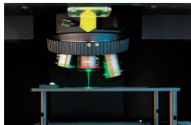
顕微レーザーラマン分光装置の試料室。形状・状態問わず微量サンプルの分析が可能。
